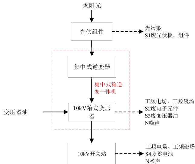
图 4 本项目运营期工艺流程图及产污环节图
