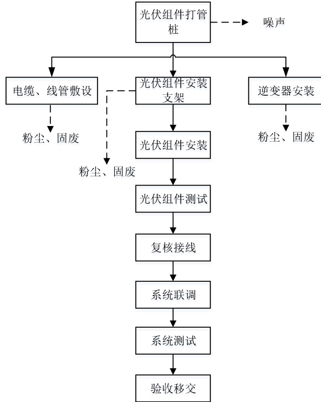
图2 光伏场区施工工艺流程及产污环节图
