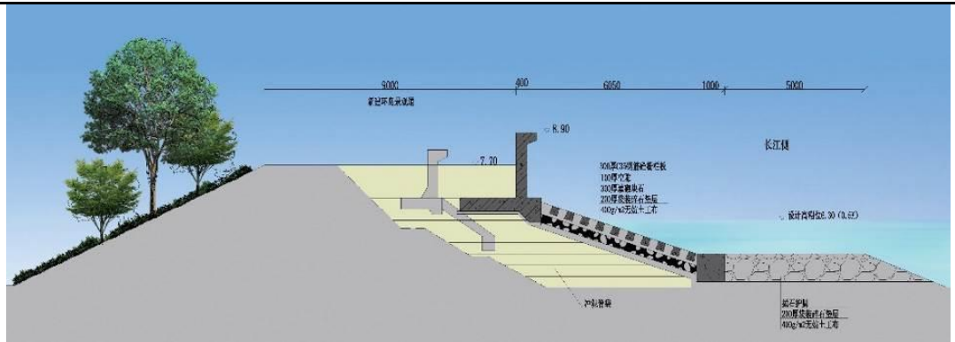
图 31 方案一：向外海侧培厚
