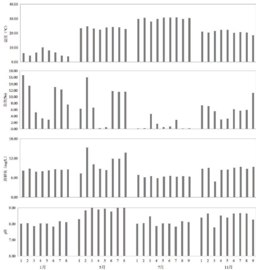
图 3.2-31 2021 年调查区域潮沟水体物理参数
