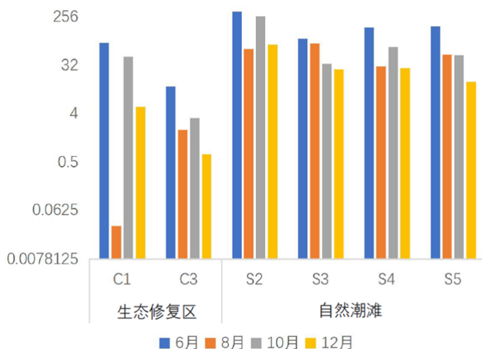
图 3.2-13 2020 年调查区域底栖生物生物量 单位: g/m 2
