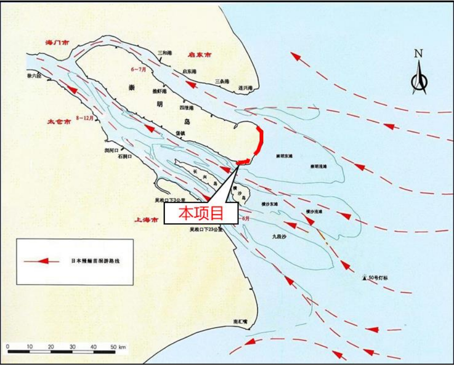
图 3.2-26 日本鳊洄游通道示意图
