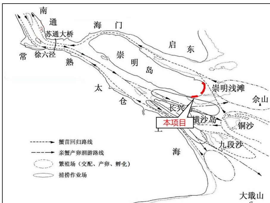
图 3.2-27 中华绒鳌蟹产卵洄游示意图
