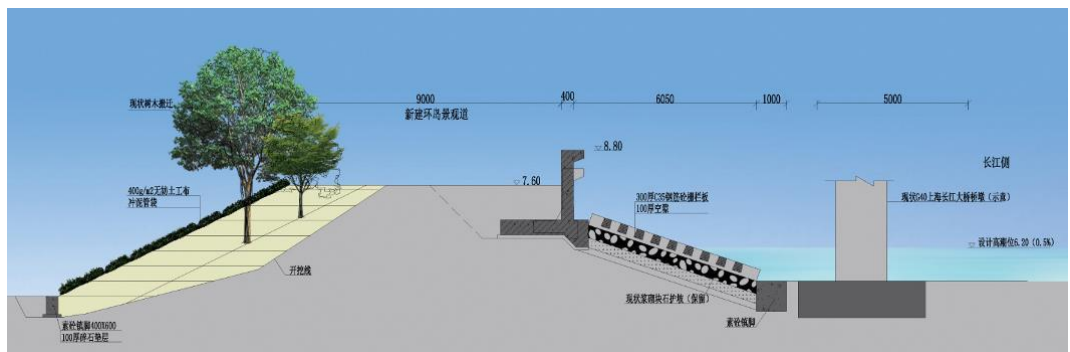
图 32 方案二：向内坡侧培厚
