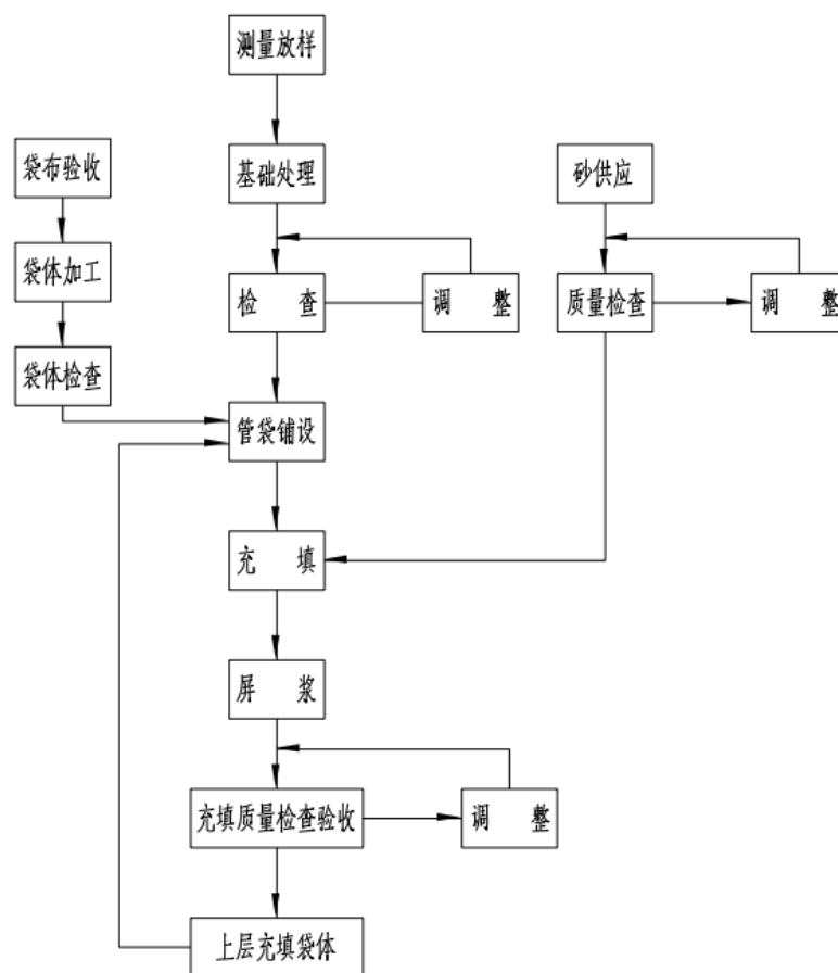
图 25 充泥管袋施工流程图
