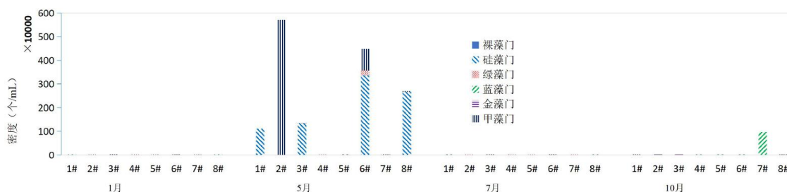
图 3.2-38 2020 年调查区域浮游植物密度分布图
