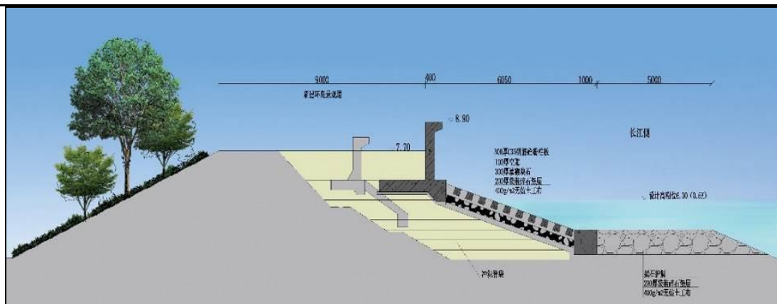
图 11 向外培厚断面示意图
