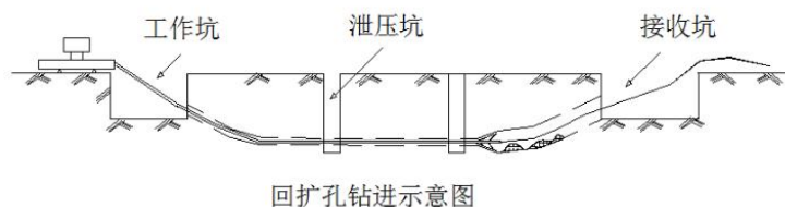
图 2-3 回扩孔钻进示意图
