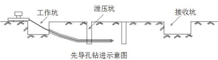
图 2-2 先导孔钻进示意图
