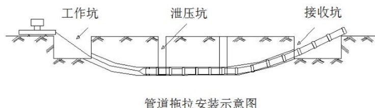
图 2-5 管道拖拉安装示意图
