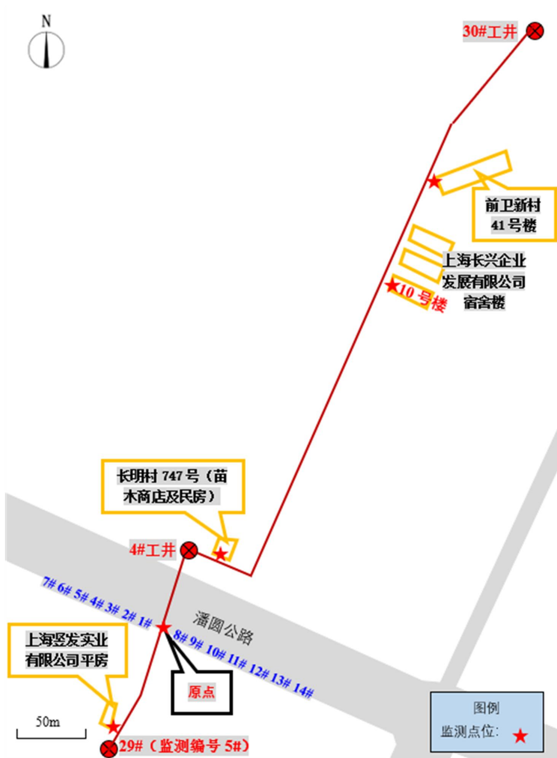
图 4.3-1 地下电缆类比监测断面示意图
