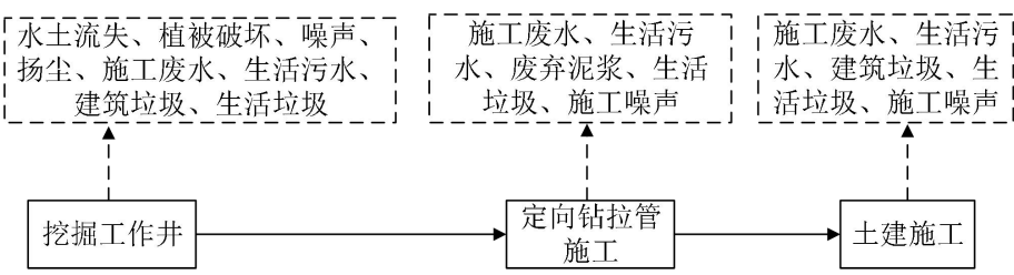
图 4-2 非开挖施工工艺流程及产污节点图
