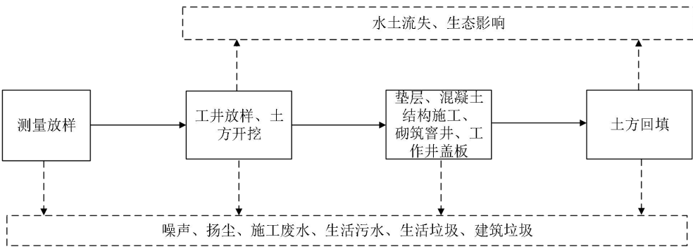
图 4-3 工井施工工艺流程及产污节点图
