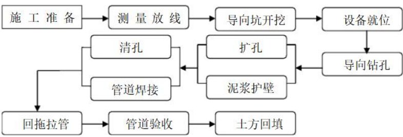
图 2-1 定向钻施工工艺流程
